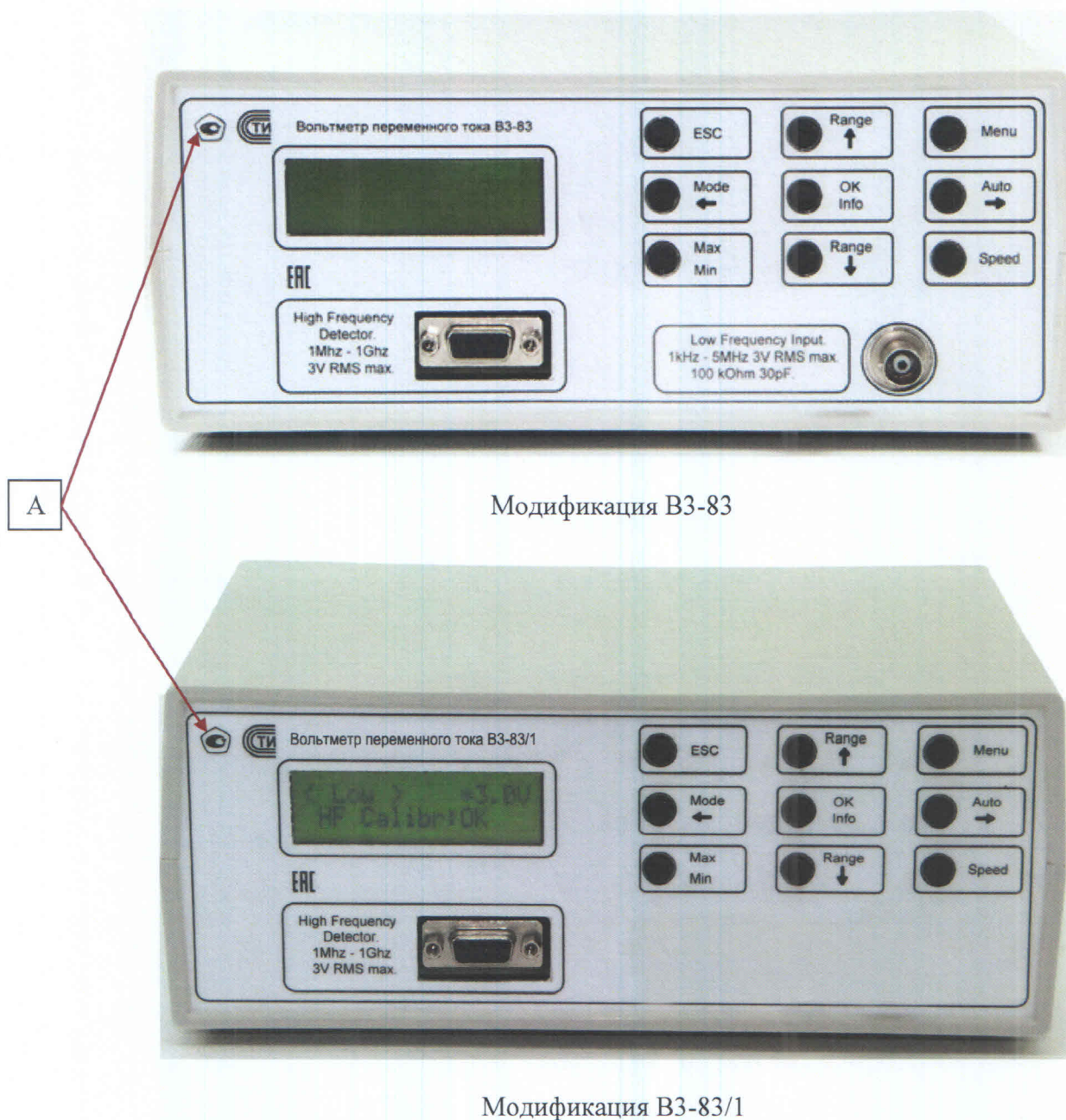
Рисунок 1 – Общий вид вольтметров и место нанесения знака утверждения типа (А)
